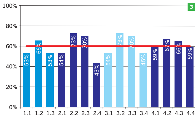
RYS. 3. Projektowe obciążenie cieplne pomieszczeń po termomodernizacji w wariantie 1 jako procent obciążenia początkowego z zaznaczeniem wartości średniej dla budynku wynoszącej 60%;
